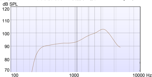
誘導コイル入力 周波数特性（磁界の強さ 31.6mA/m）
